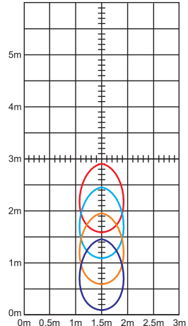
Mit min. 5lx angestrahlte Fläche bei Leuchtenhöhe(Lh)
